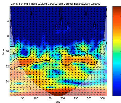
Obr.2 Krížové vlnkové výkonové spektrum MgII indexu a koronálneho indexu(03/2001-02/2002).
