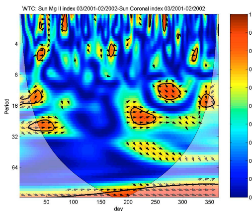
Obr.3 Vlnková koherencia MgII indexu a koronálneho indexu (03/2001-02/2002).
